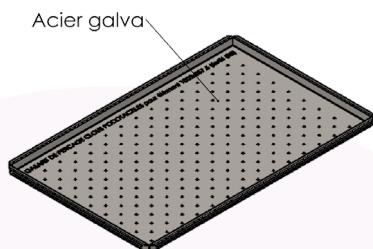
Gabarit de perçage
