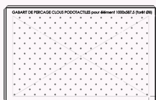
Gabarit de perçage
